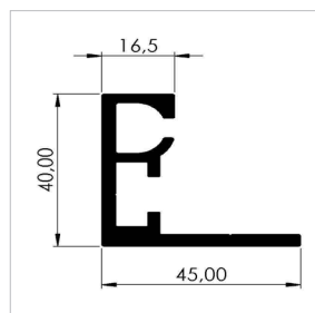
Profil Keder FRAME 45x40mm
