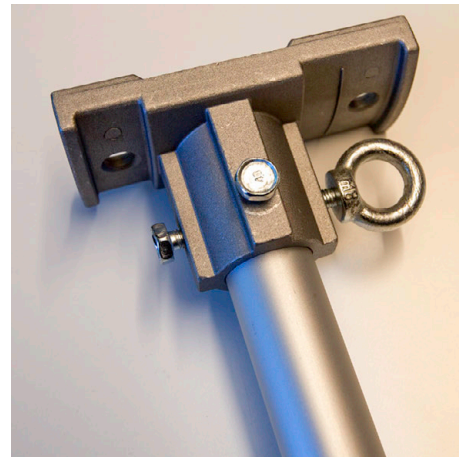
Hållaren är av gjuten metall och röret i aluminium.
